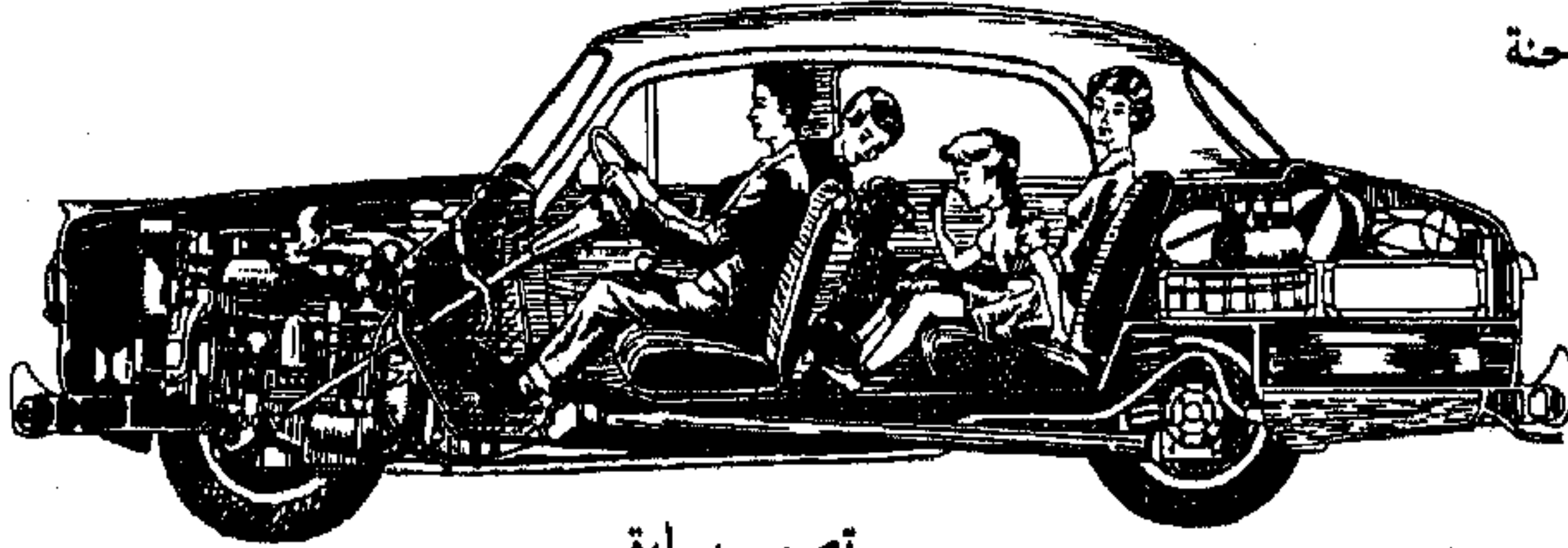
تصميم سيارة
